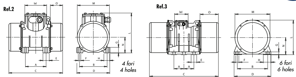
Dimensioni (mm) - Dimensional Specifications (mm)
