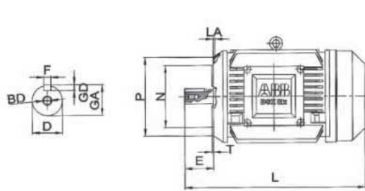
IMB14 (IM3601)
