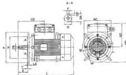
M2JA160-200
