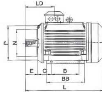
IMB34 (IM2101)
