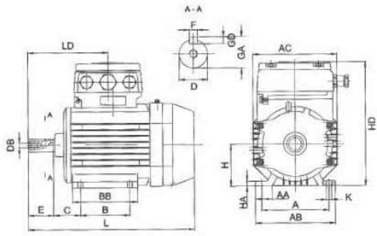
M2JA80-132
